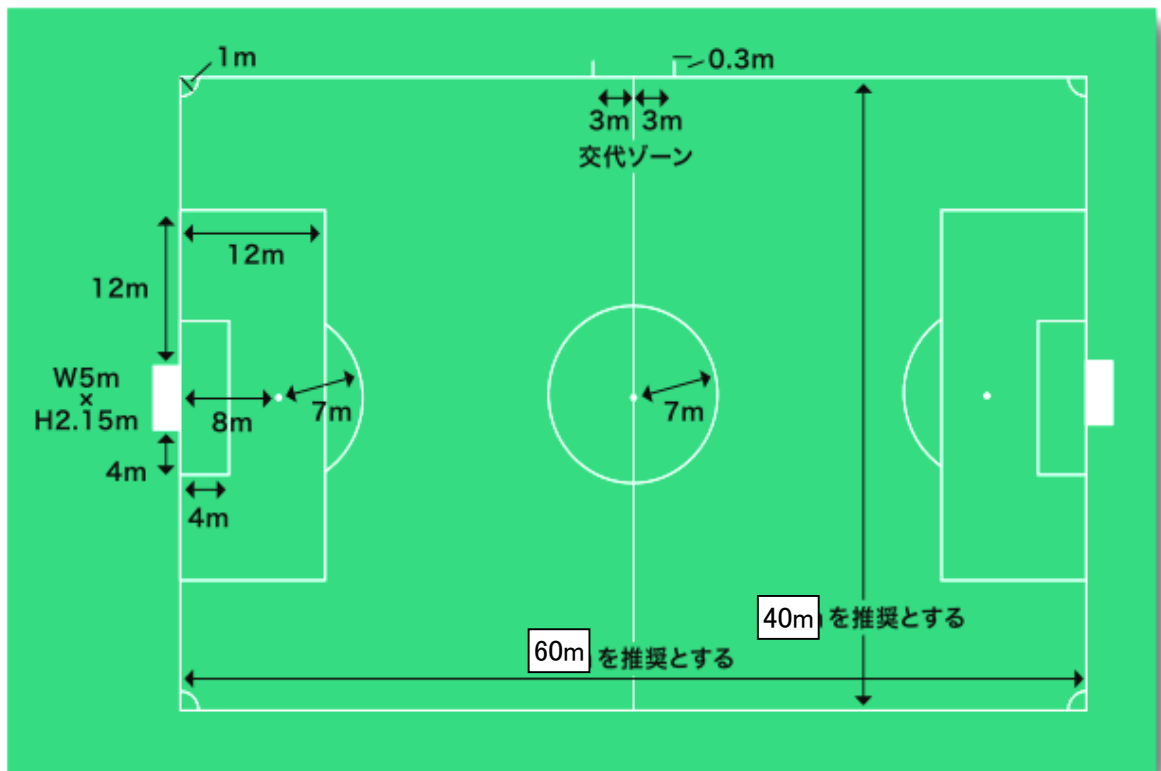
8人制サッカーフィールドレイアウト見本
